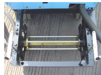
ブレード軸2分割
