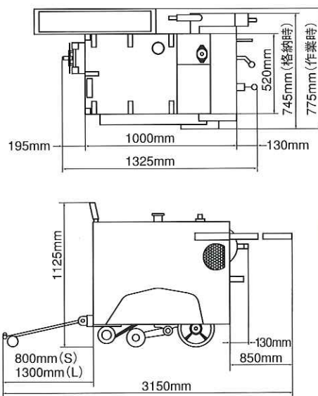
■概略寸法
