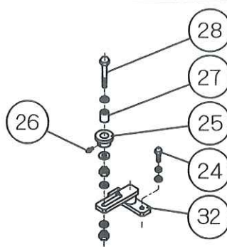
縦軸アウター～デフ
