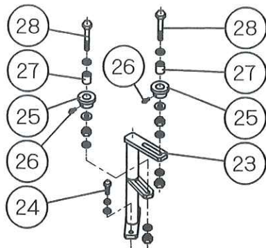
減速機～縦軸アウター
