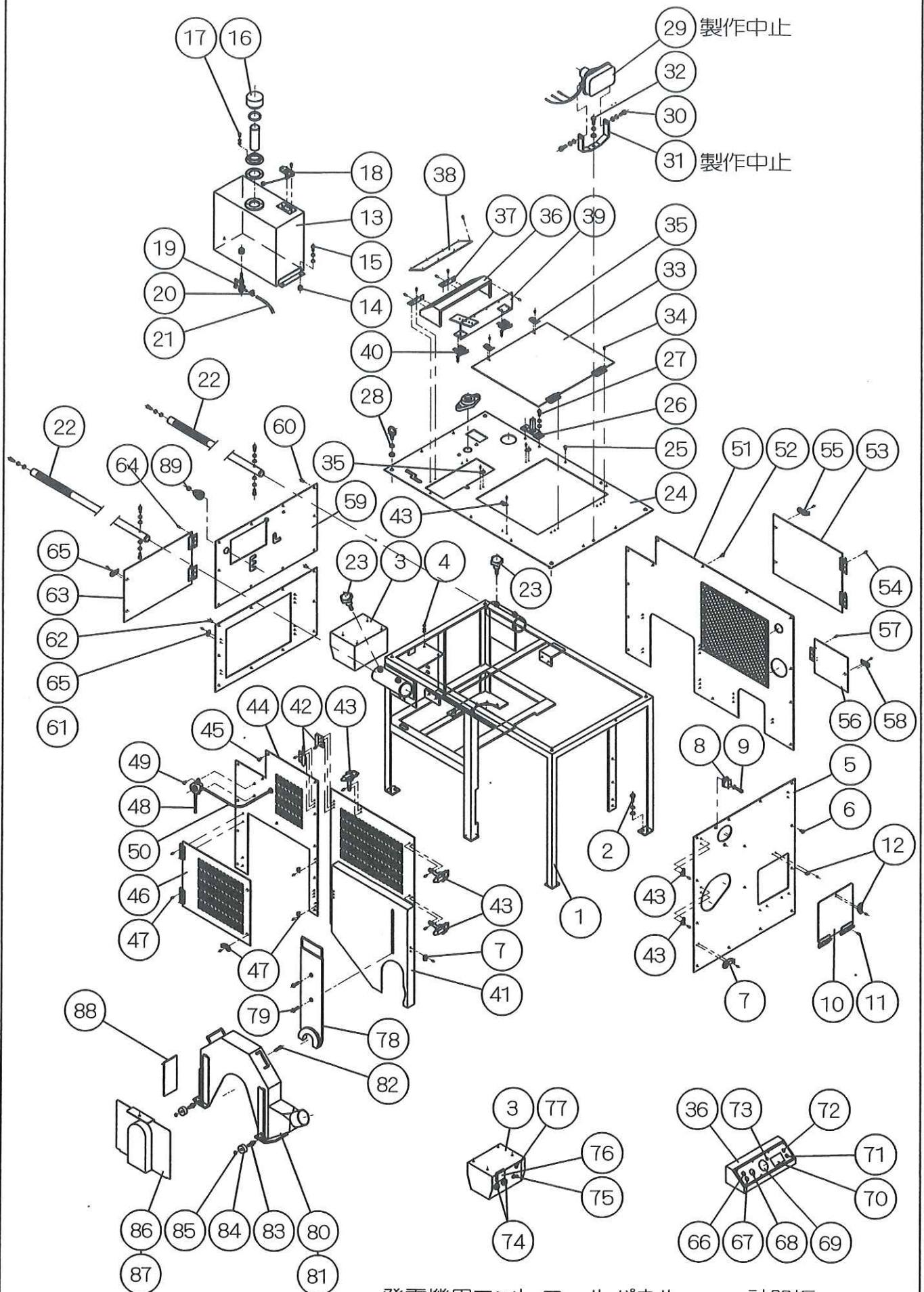
発電機用コントロールパネル
